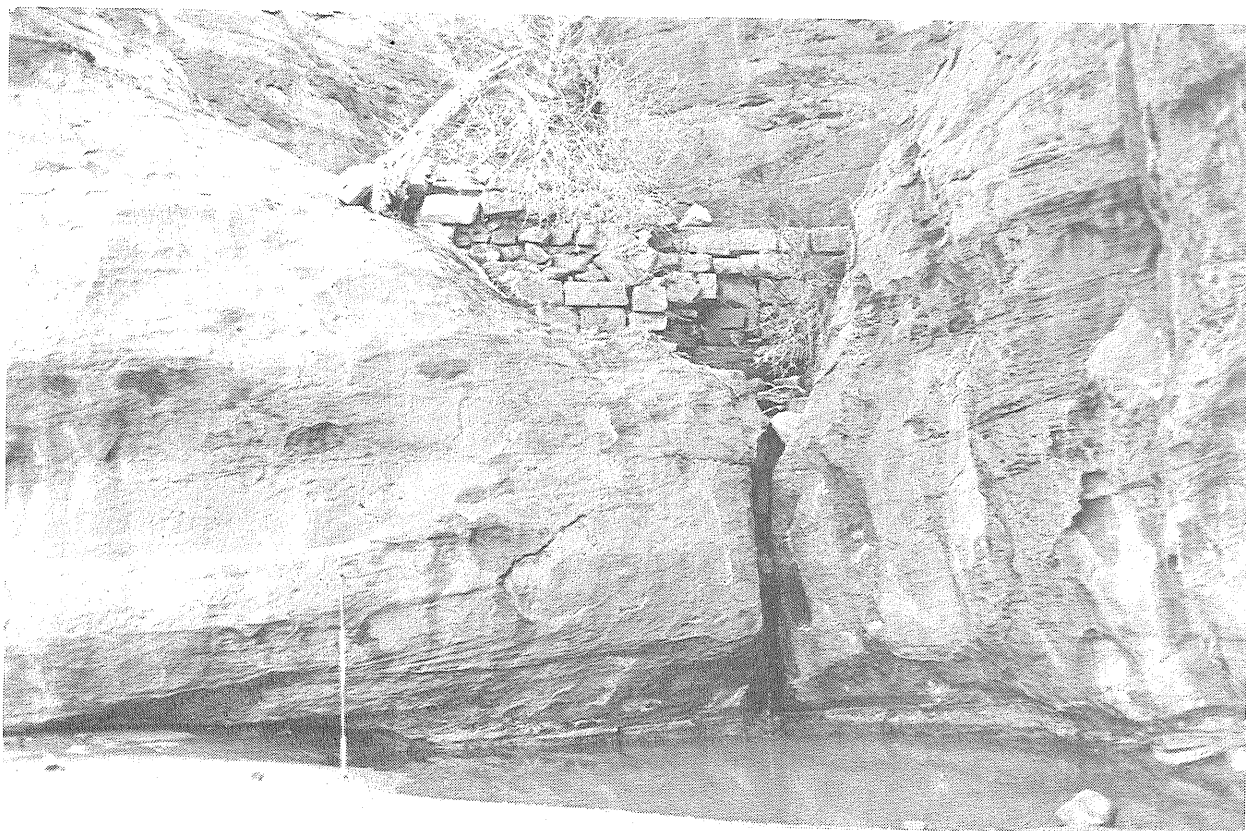
Pl. XXXIX, 2: Sed 'Um Darag (Wadi Barah): Nabataean Dam.
